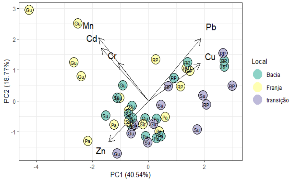
Gráfico 1: Distribuição de Mn, Cd, Cr, Pb, Cu e Zn em locais diferentes na CEP
