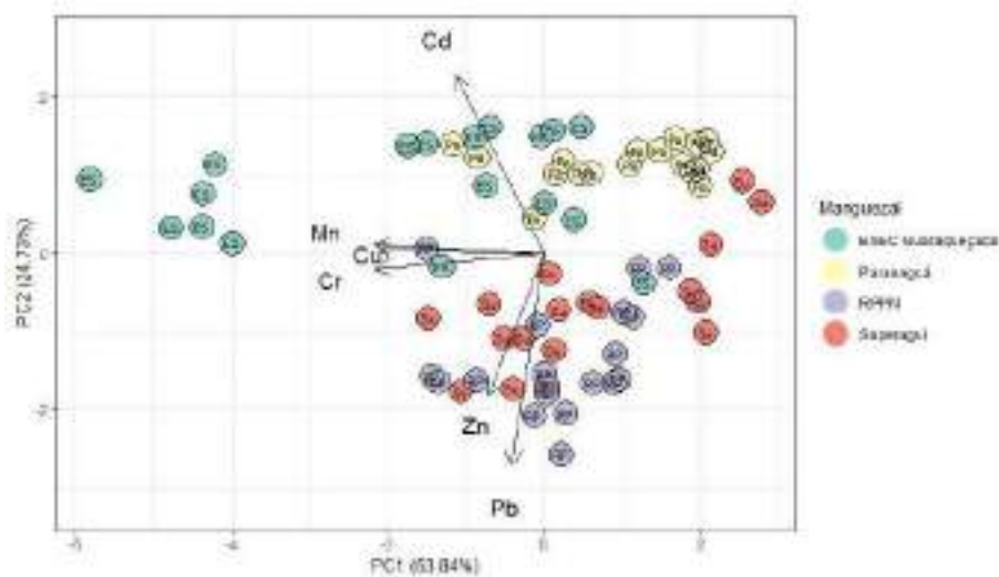
Gráfico 2: Distribuição de Mn, Cd, Cr, Pb, Cu e Zn nos diferentes manguezais analisados no CEP
